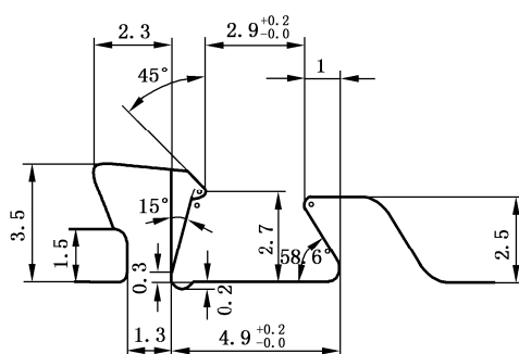
图 C.1 穿条型材槽口示意图
